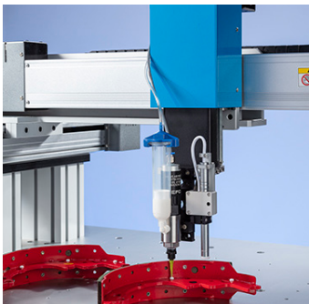
725D 安装在 GV 点胶平台上为汽车制动钳点涂润滑脂。
