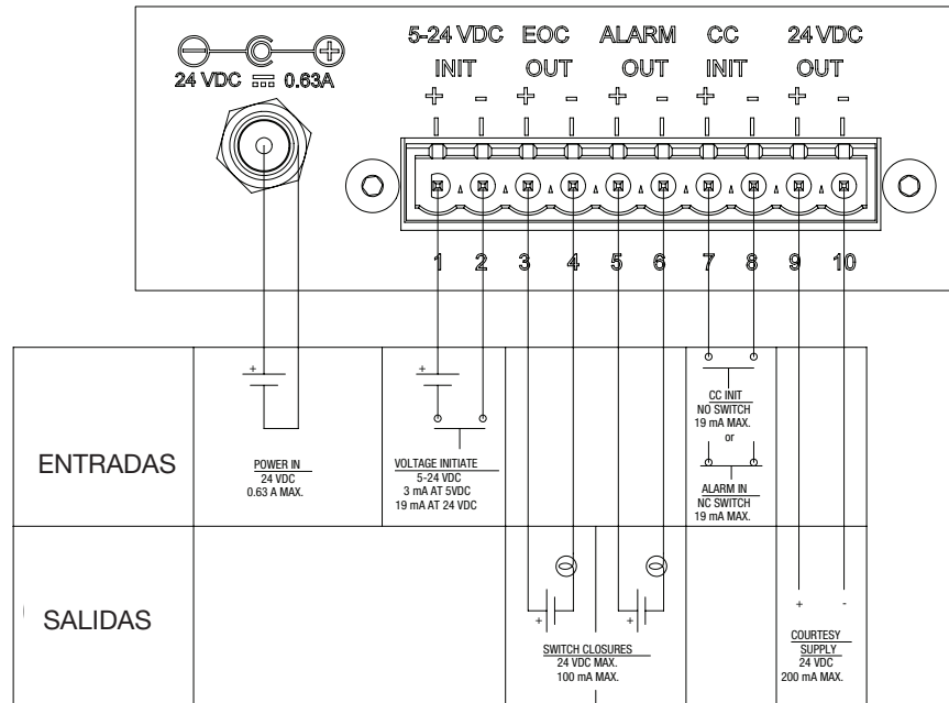
Diagrama de Alambrado Externo de E/S
