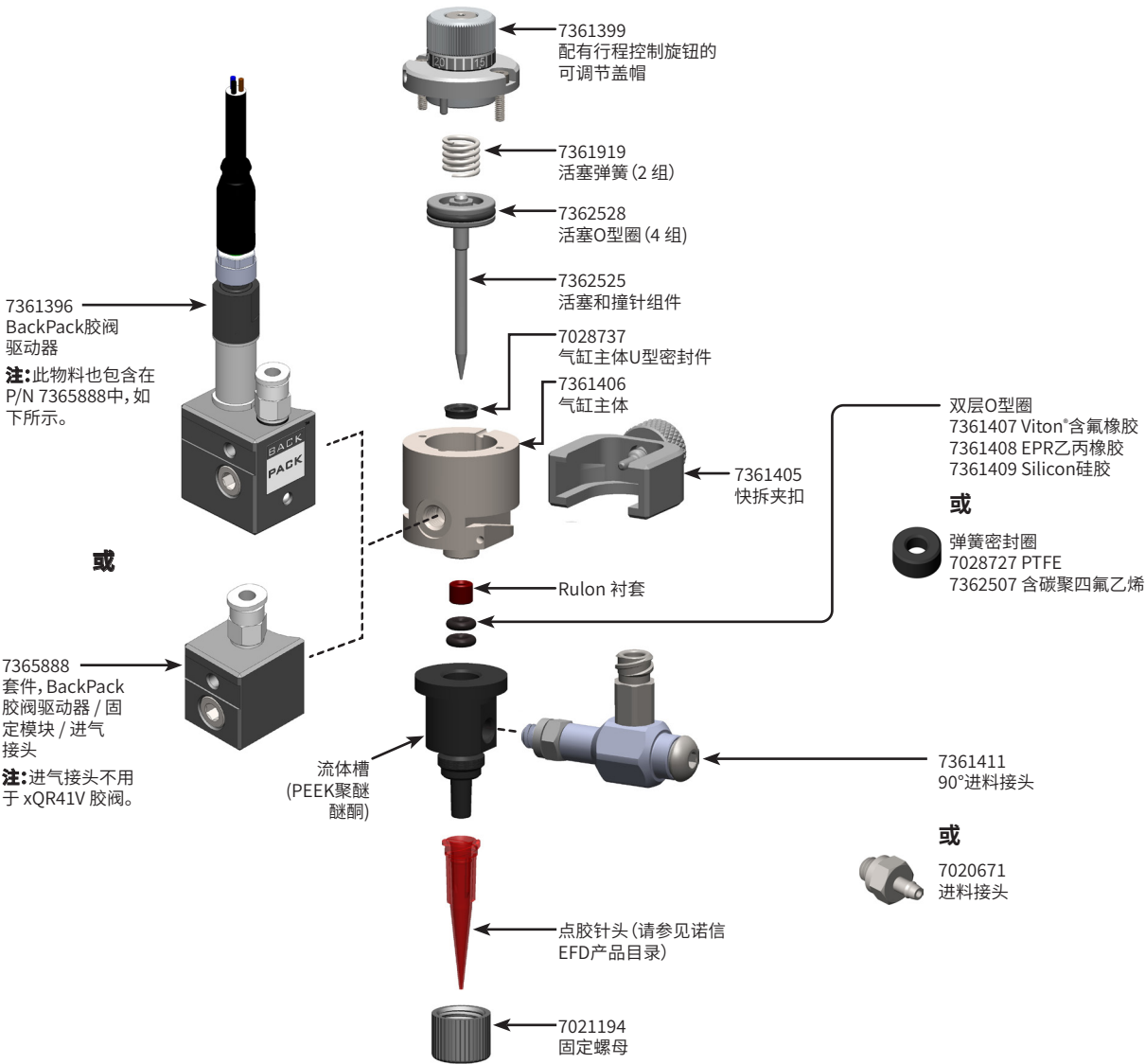
xQR41V胶阀可更换部件 (如图所示为配有双层O型圈的胶阀)
