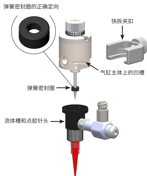
为配有弹簧密封圈的胶阀更换流体槽
