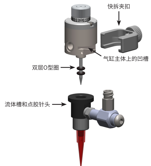
为配有双层O型圈的胶阀更换流体槽
