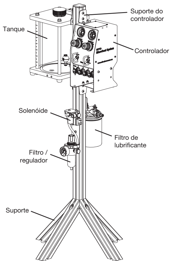
Sistema típico MicroCoat montado sobre um suporte
