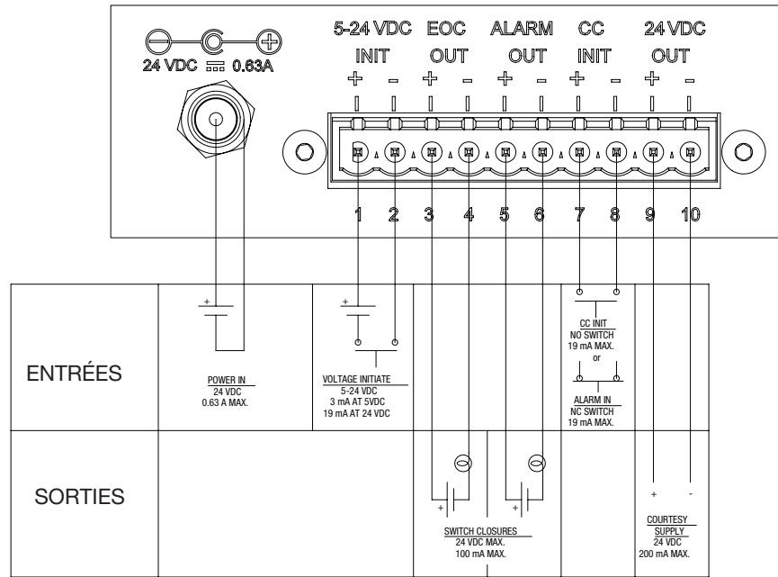
Schéma de câblage externe E/S
