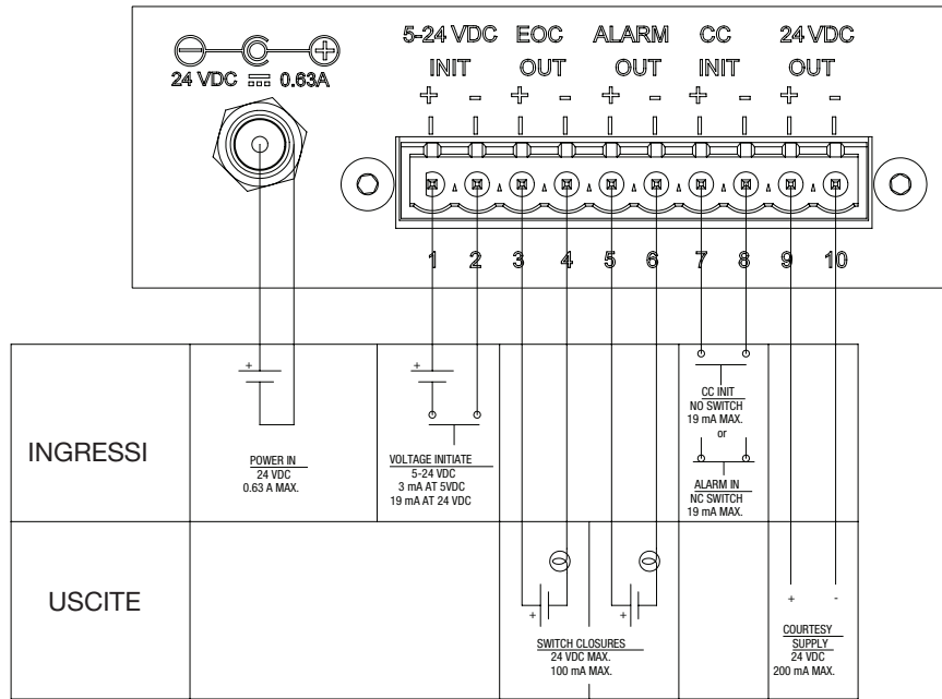
Schema di cablaggio I/O esterni
