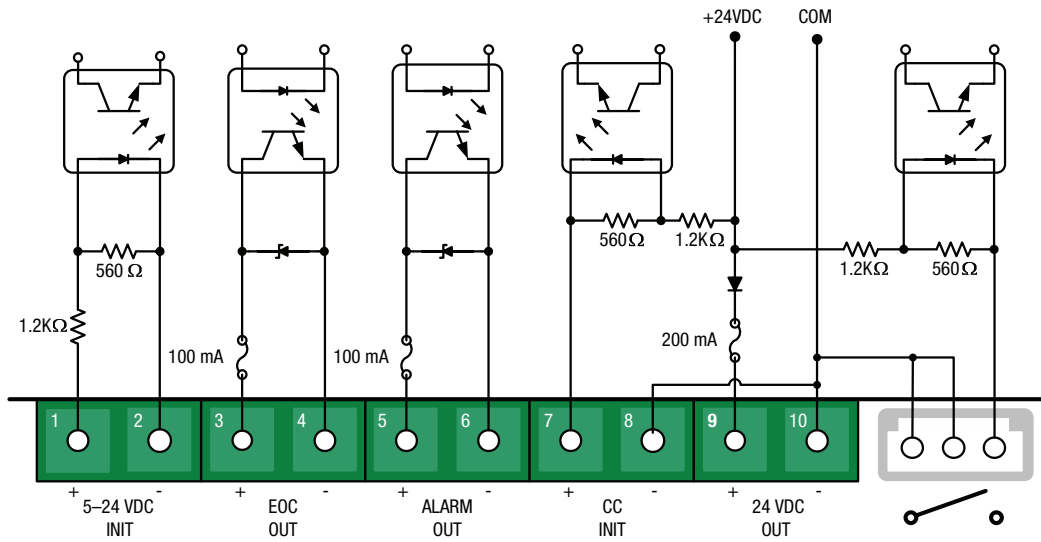
I/O Elektrischer Schaltplan
