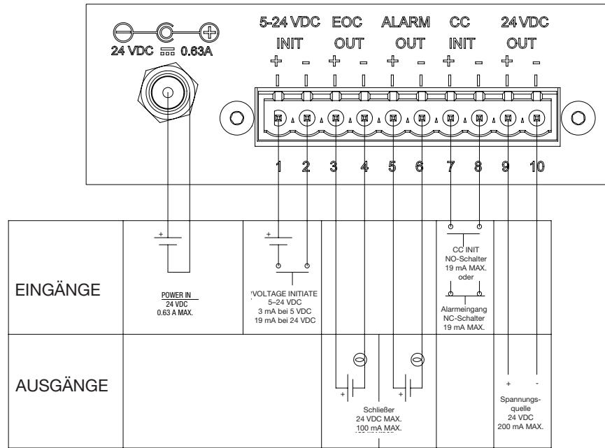
I/O Externer Anschlussplan
