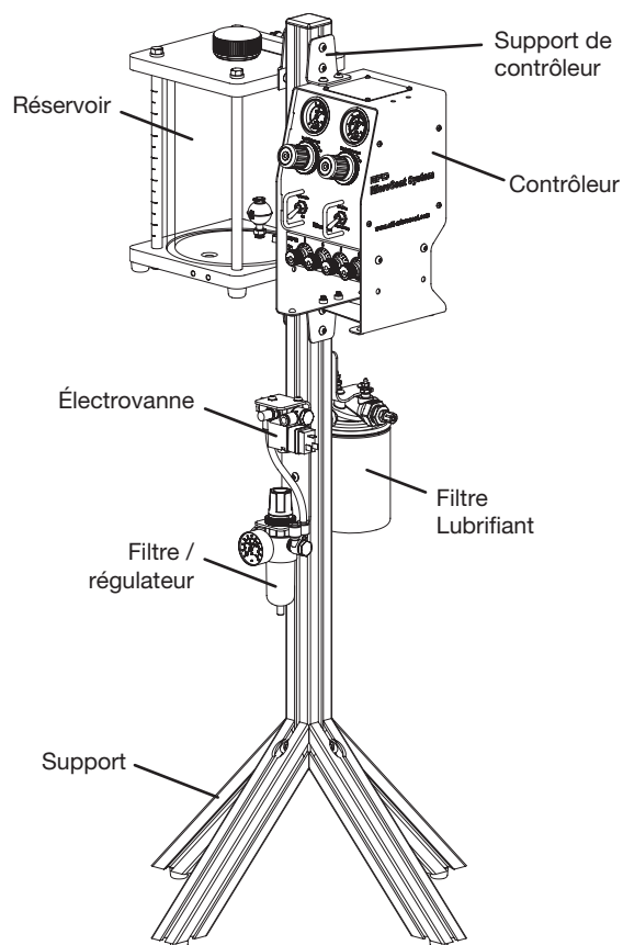
Système MicroCoat type monté sur un pied
